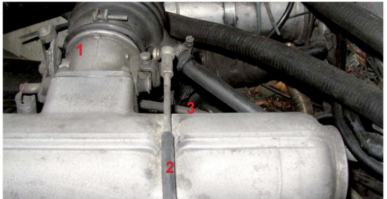
Ansaugkrümmer: 1 Klappenstutzen 2 Stupsgestänge 3 Unterdruckleitung zur ESP
