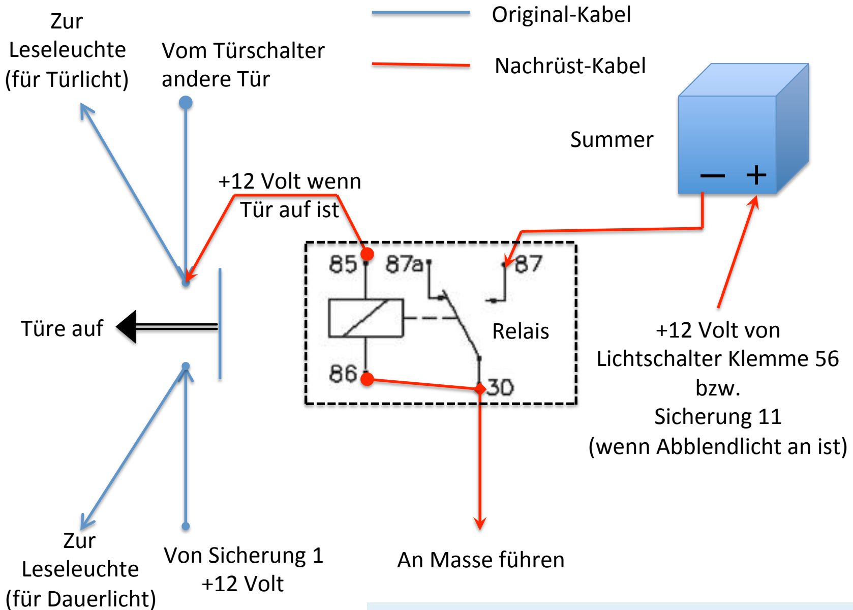
Relaisschaltung für Aktivierung Lichtwarn-Summer über Türkontaktschalter im W114/W115
